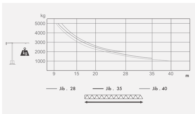
Lastdiagramm
